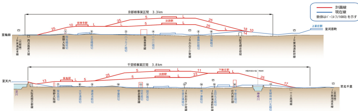
計画略図
